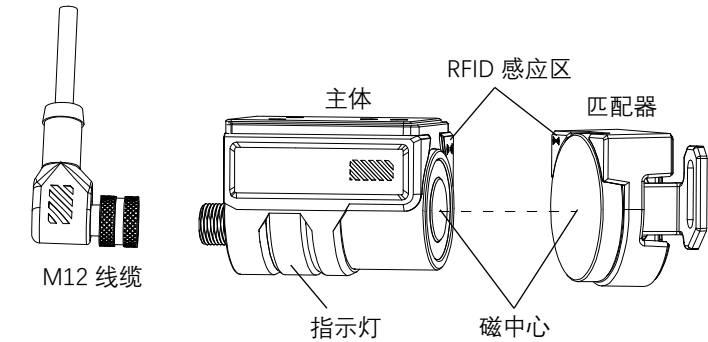
图 5-1 安全门开关构成图
