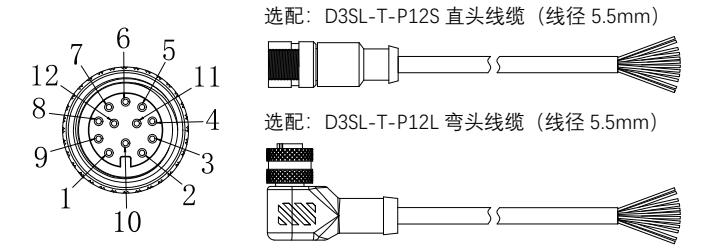
图 7-1 M12 插头线缆线序图
