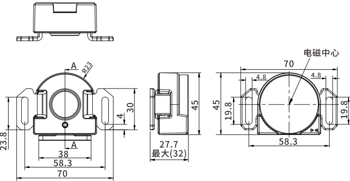
图 5-2 匹配器尺寸图
