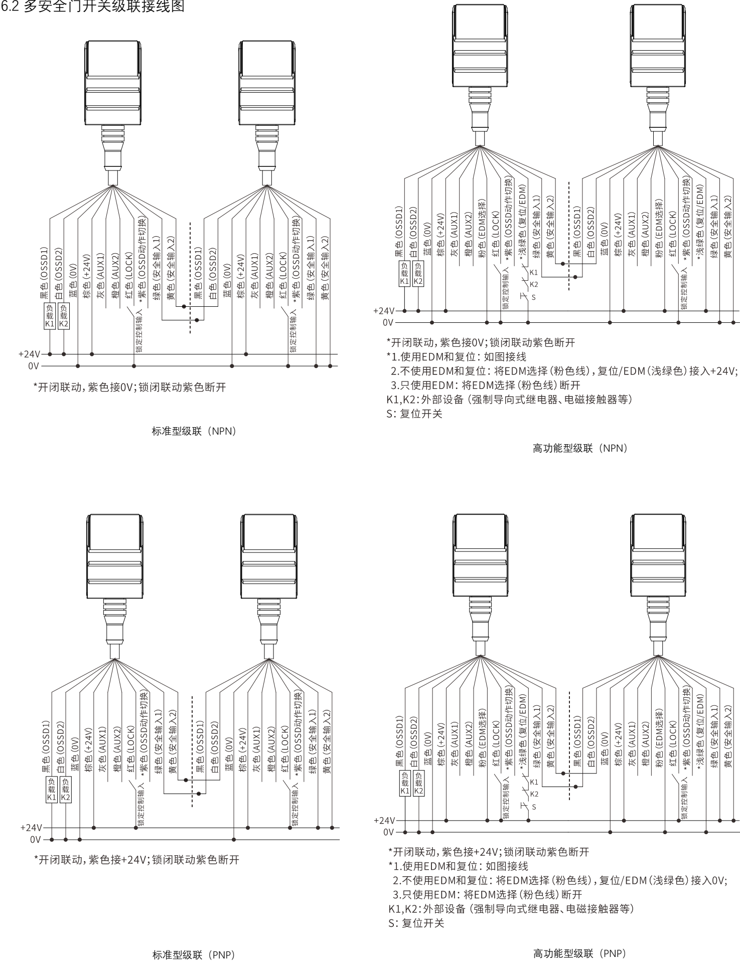
图 6-2 多安全门开关级联接线示意图
