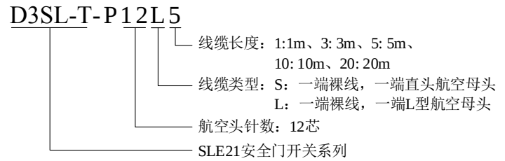
图 7-2 线缆型号说明示意图
