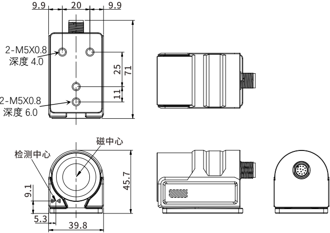
图 5-3 主体尺寸图
